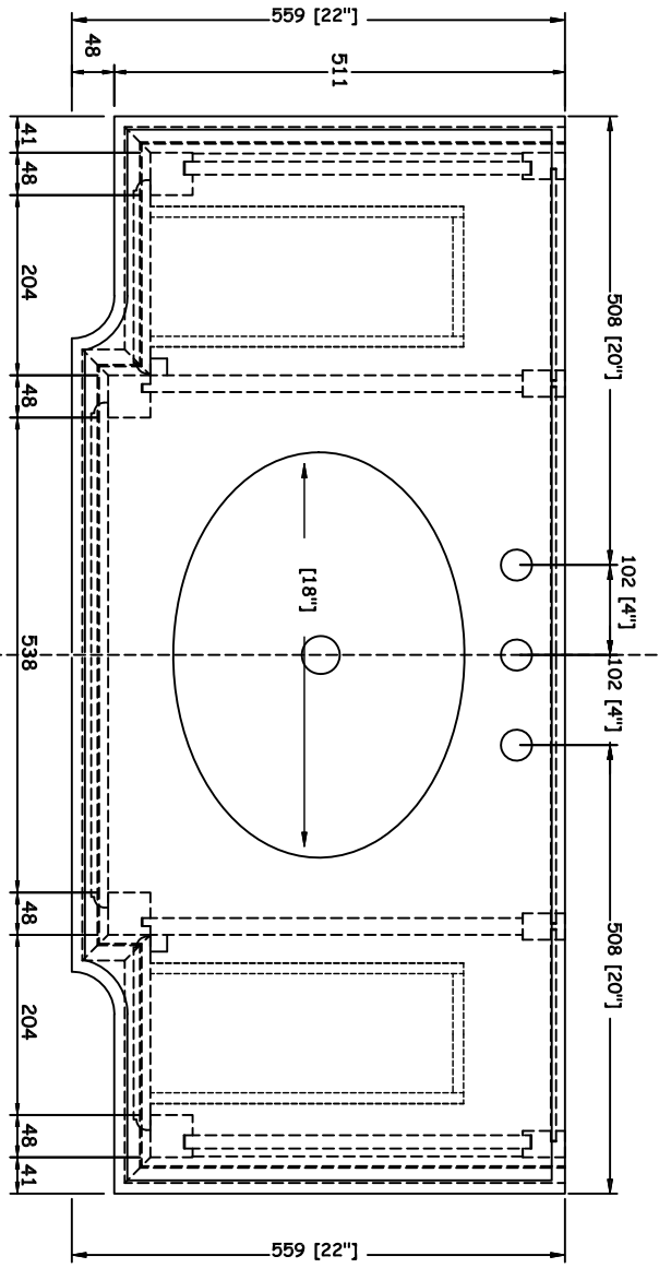
Lana-48 洗手台 SIZE: 1220*559*876mm
